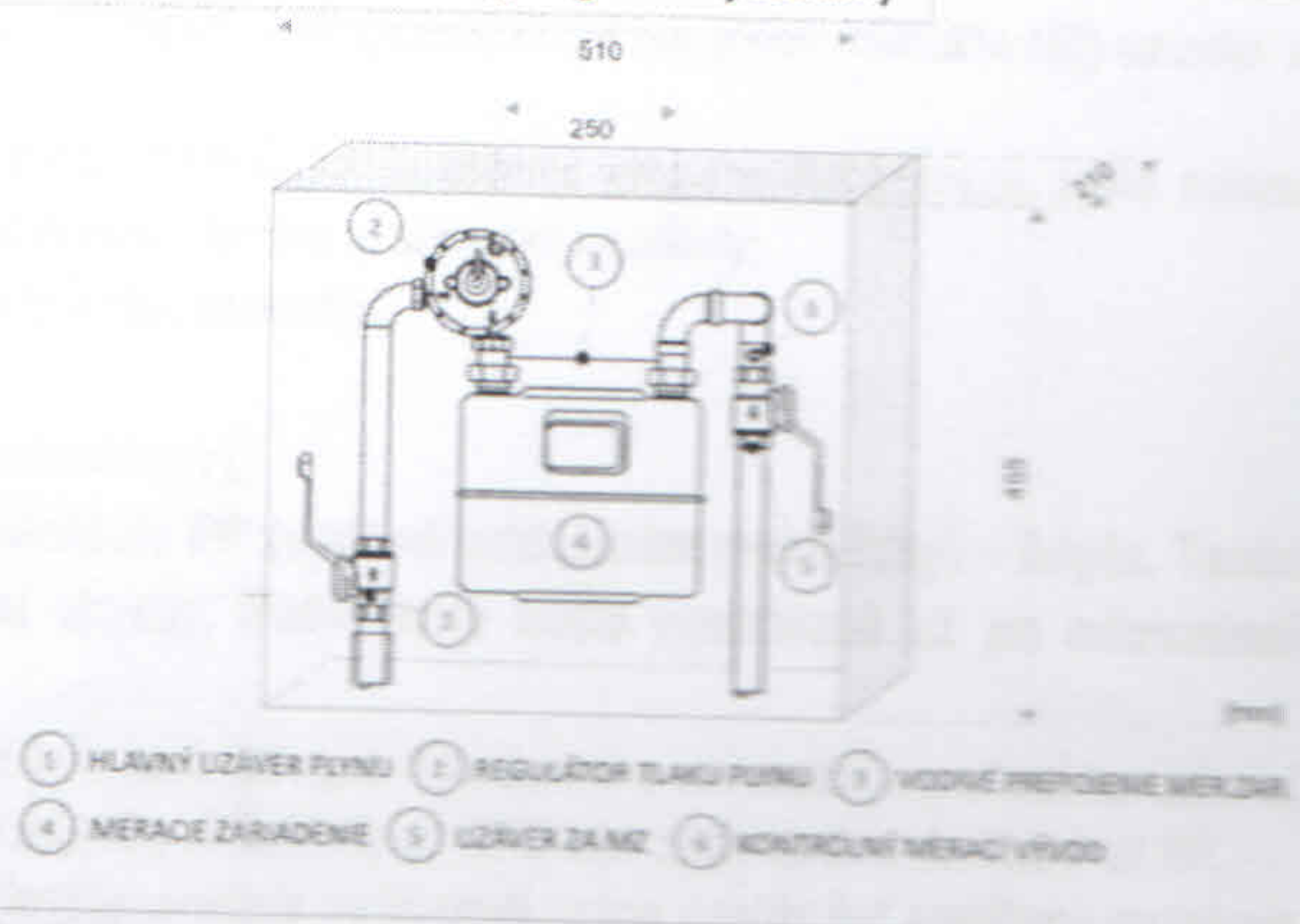
Detail meracej (domovej) regulačnej zostavy
