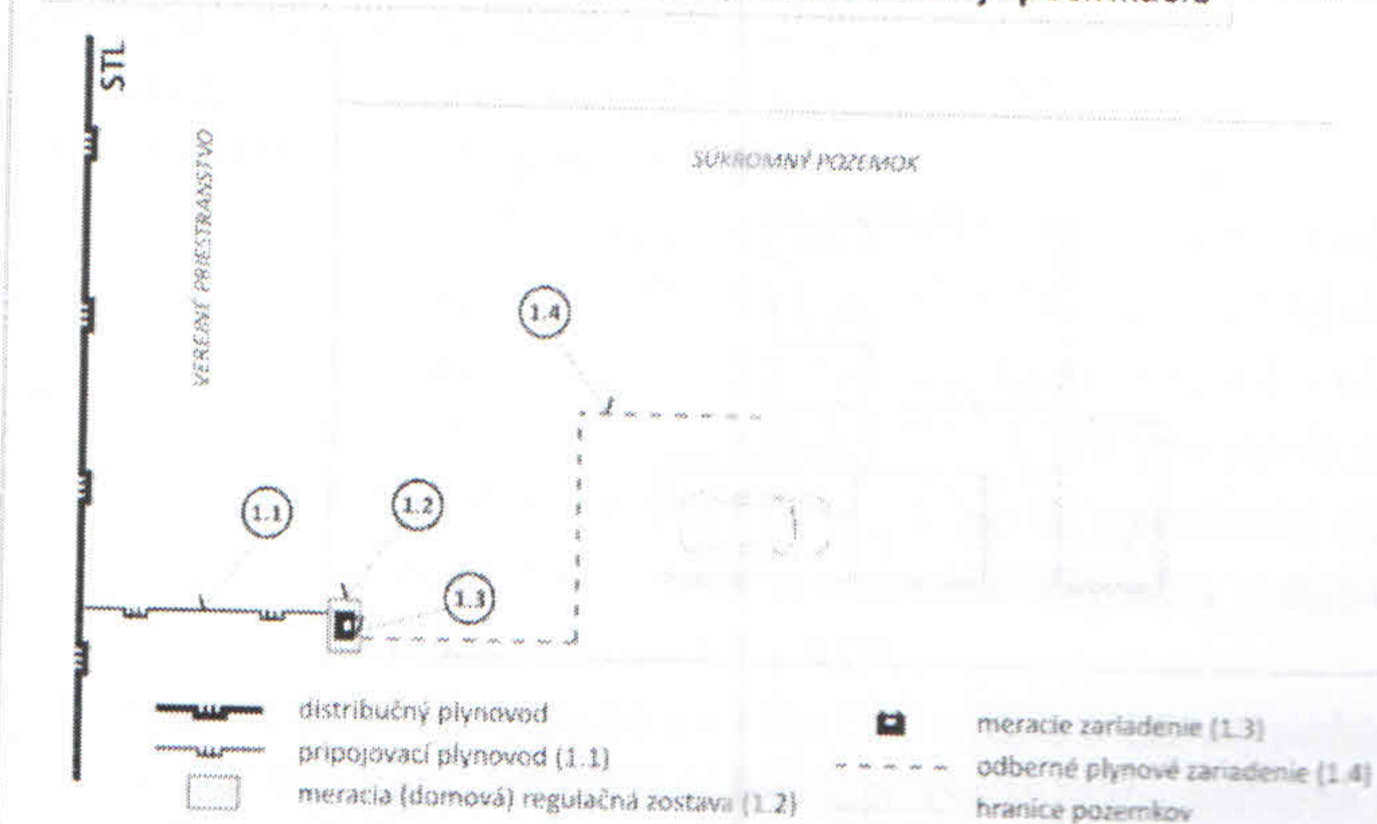
Orientačný náčrt zariadení podľa vyššie uvedenej špecifikácie
